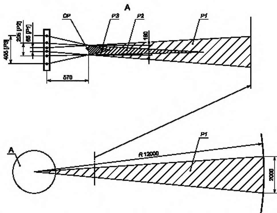
P1 — ширина неосвещаемой зоны при расстоянии между лампами 65 мм; P2 — ширина неосвещаемой зоны при расстоянии между лампами 205 мм; P3 — ширина неосвещаемой зоны при расстоянии между лампами 405 мм
