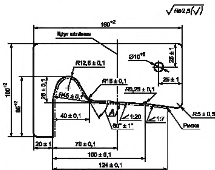
Рисунок Б.1 — Профиль обода колеса
