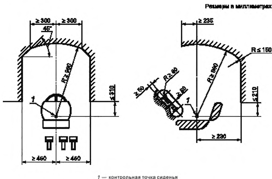
Рисунок 7 — Размеры внутреннего пространства кабины
