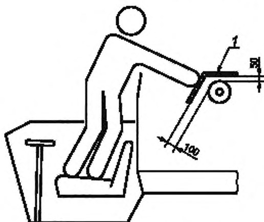
Рисунок 9 — Доступ к распределительному шнеку
