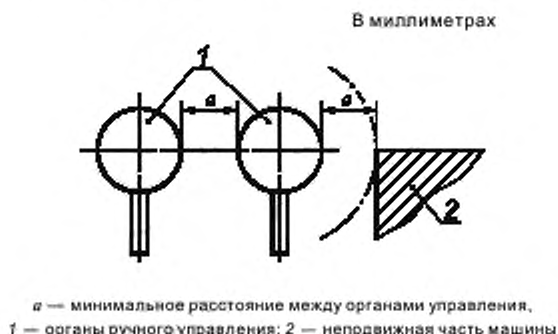
Рисунок 1 — Расстояние между органами управления
