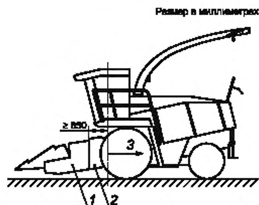
f — жатка; 2 — кожух подающего аппарата; 3 — зона дополнительного контроля (за пунктирной линией)
