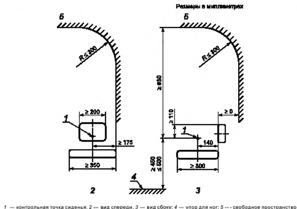
Рисунок 3 — Размеры сиденья инструктора
