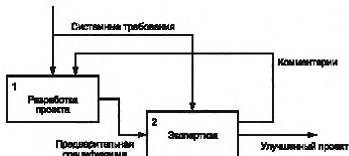
Рисунок В.5 — Пример обратной связи
