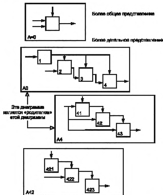
Рисунок В.2 — Структура SADT-модели: декомпозиция диаграмм
