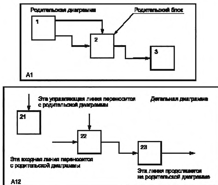
Рисунок В.4 — Взаимосвязь диаграммы A12 с родительской диаграммой A1
