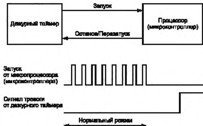
Рисунок А.12 — Структурная схема и временные диаграммы модуля временного и логического контроля последовательности выполнения программ
