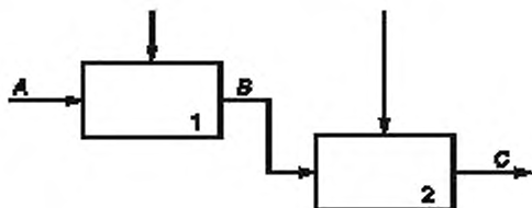
Рисунок В.11 — Последовательная связанность
