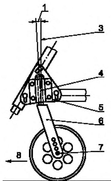
а) Узел самоориентирующегося колеса, продольная плоскость
