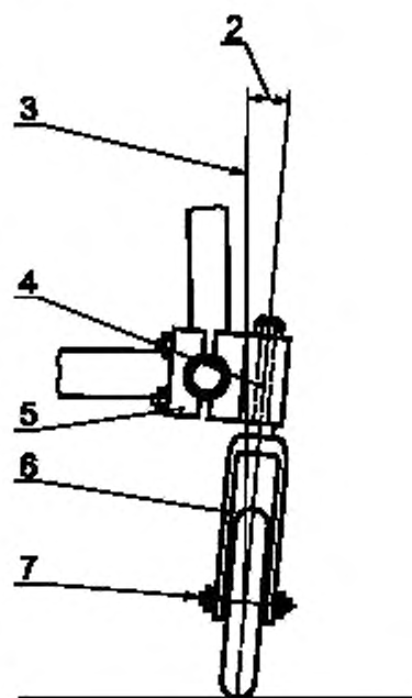
б) Узел самоориентирующегося колеса, поперечная плоскость
