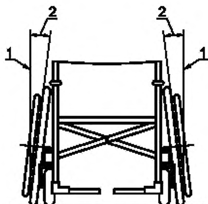
1 – вертикаль; 2 – отрицательный развал колес
