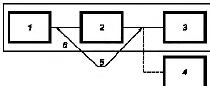
1 — источник излучения, стабилизированный из состава РЭСМ на 0,85; 1,31; 1,49; 1,55; 1,625 мкм; 2 — аттенюатор оптический; 3 — ваттметр из состава РЭСМ; 4 — поверяемый ваттметр; 5 — волоконно-оптический кабель; 6 — РЭСМ
