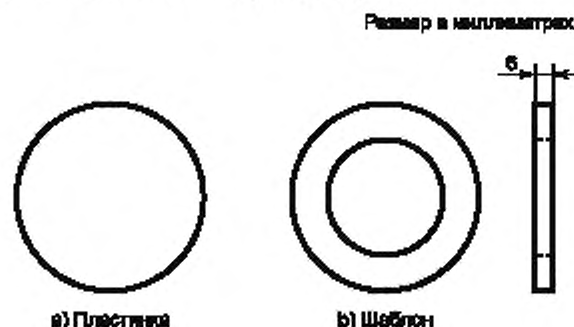
Рисунок 2 — Приспособления для испытаний на проницаемость
