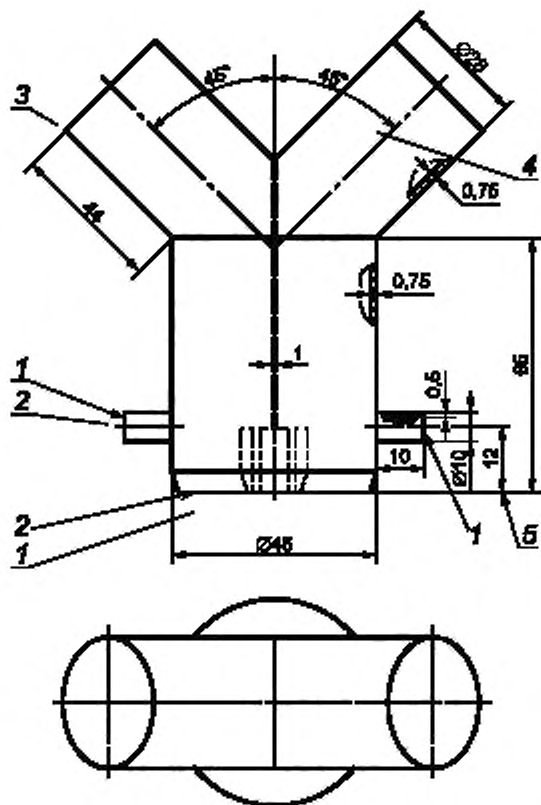
1 — выходной патрубок тройника; 2 — штуцер для присоединения тягонапомера; 3 — патрубок, направленный к линии выдоха ИП; 4 — патрубок, направленный к линии вдоха ИП; 5 — штуцер для установки термоэлектрического преобразователя
