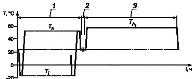
1 — первый этап испытаний; 2 — второй этап испытаний; 3 — третий этап испытаний; T_n — температура выдержки, равная (53,0 \pm 1,0)^\circ\text{C} ; T_{n2} — температура выдержки, равная (58,0 \pm 0,5)^\circ\text{C} ; T_l — температура выдержки, равная минус (18,0 \pm 2,0)^\circ\text{C}
