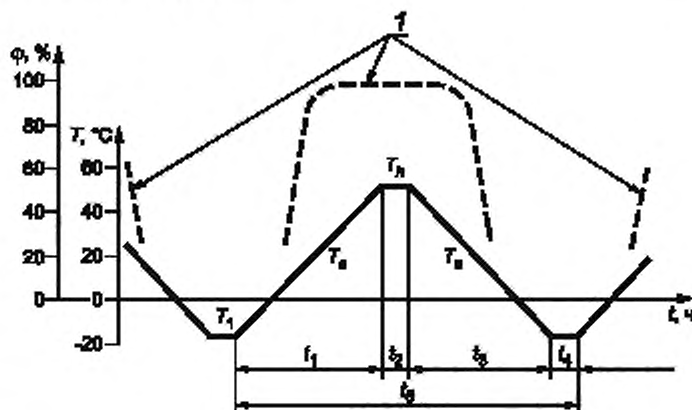
\varphi — относительная влажность в течение температурного цикла; T_n — температура выдержки, равная (53,0 \pm 1,0)^\circ\text{C} ; T_l — температура выдержки, равная минус (18,0 \pm 2,0)^\circ\text{C} ; T_g — перепад температур, равный (14 \pm 2,0)^\circ\text{C} в течение часа; t_1 — t_5 — интервалы времени; \varphi — влажность
