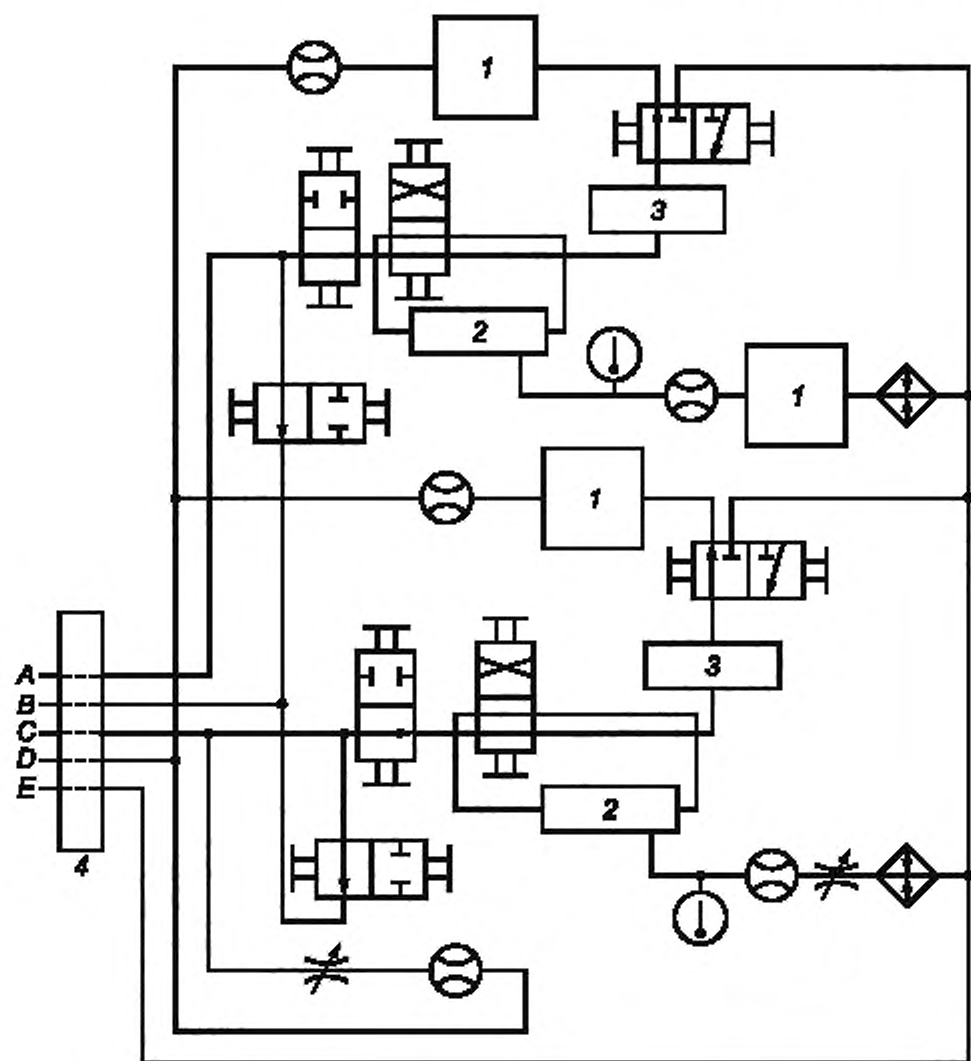
1 — регулятор расхода; 2 — смеситель; 3 — датчик АСЧ; 4 — подключение к испытательному стенду; А — отбор пробы выше по потоку; В — гидробак с испытательной жидкостью; С — отбор пробы ниже по потоку; D — к насосу; E — насос для жидкости при разбавлении пробы
