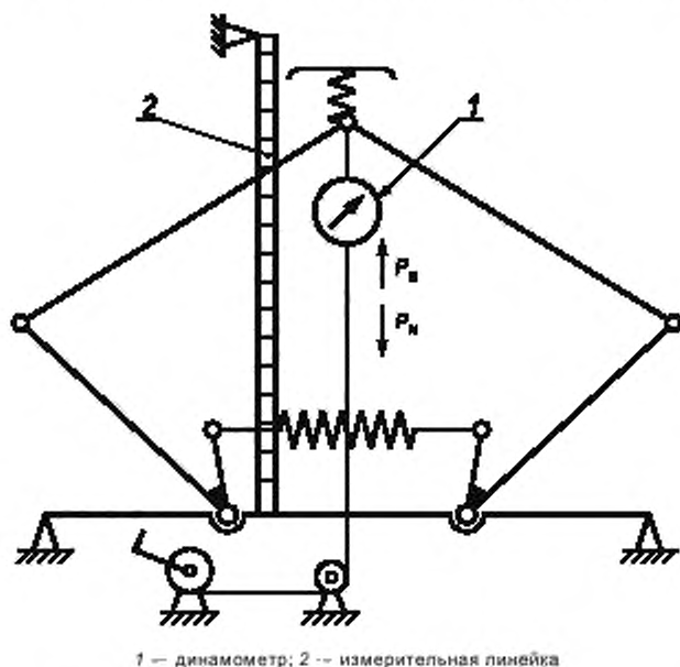
Рисунок 2 — Кинематическая схема для снятия статической характеристики
