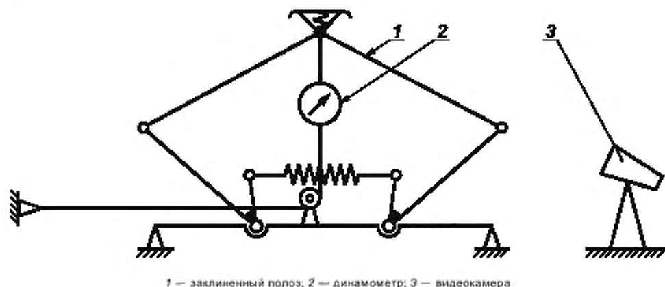
Рисунок 10 — Схема для определения вертикальной составляющей аэродинамической силы
