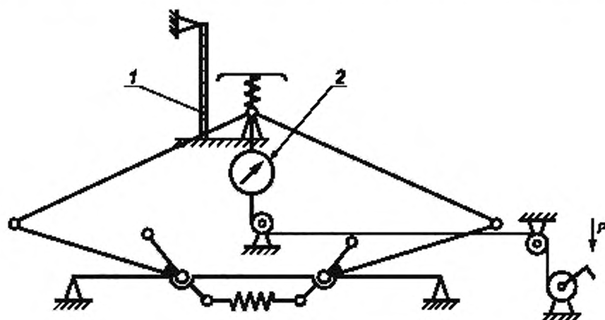
Рисунок 7 — Кинематическая схема для определения жесткости кареток
