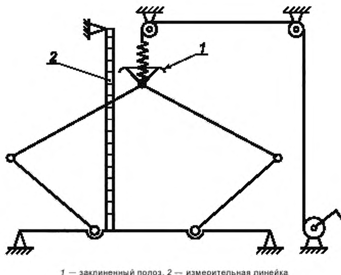
Рисунок 4 — Кинематическая схема для определения приведенной массы
