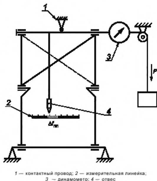
Рисунок 5 — Кинематическая схема для определения поперечной жесткости
