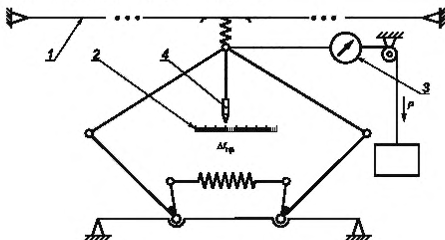
Рисунок 6 — Кинематическая схема для определения продольной жесткости
