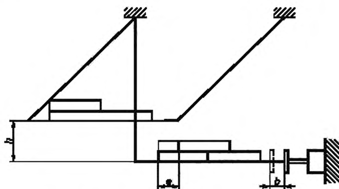
Рисунок 2 — Метод испытания маятниковым прибором
