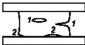
Рисунок 2 — Иллюстрация когезионного и адгезионного разрывов по всей глубине герметика
