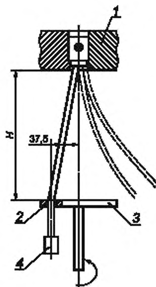
1 — панель; 2 — пильза; 3 — диск, 4 — груз
