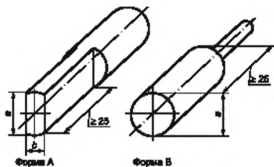
Рисунок 5 — Шупы (см. 9.2.4.5)
