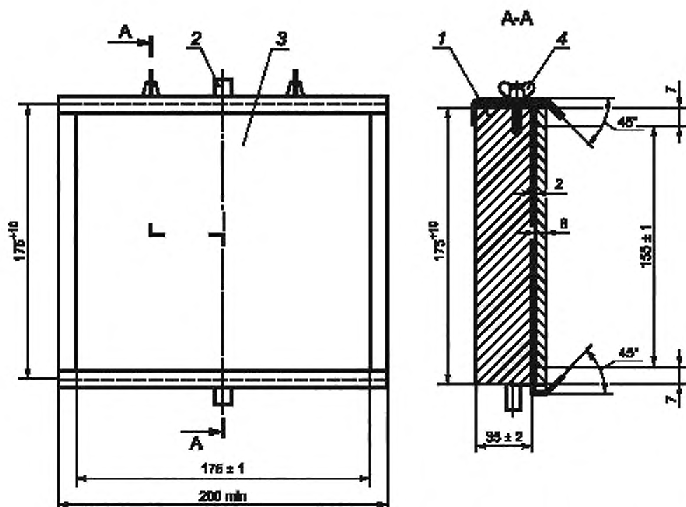
Рисунок 6 — Ударный элемент маятника для механических испытаний (см. 9.2.5.2.1)
