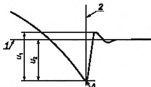
f — линия развертки; 2 — момент нулевого тока; А — начальная точка
