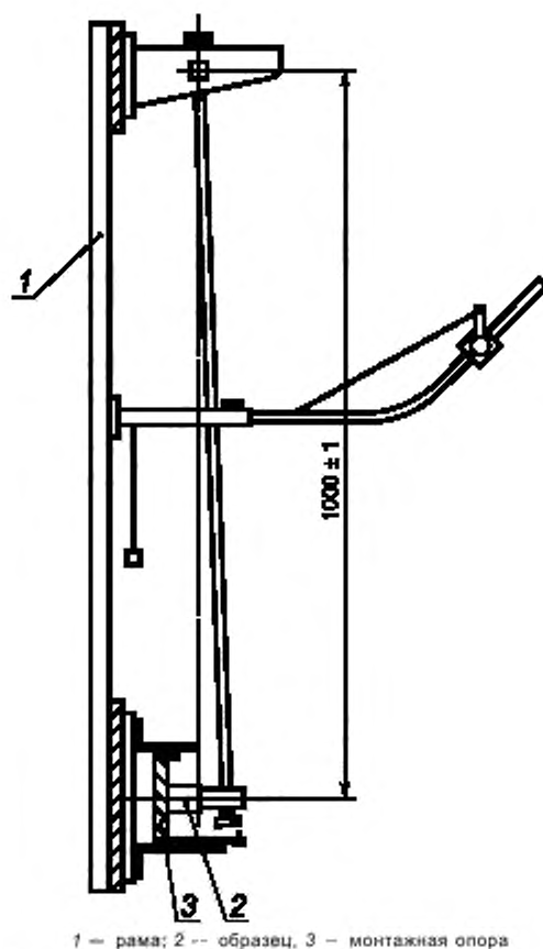
1 — рама; 2 — образец, 3 — монтажная опора Рисунок 12 — Устройство для испытаний на механический удар (9.13.2.1)
