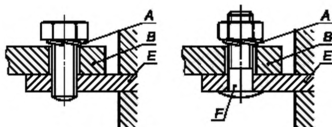
A — зажимное устройство; B — кабельный наконечник или шина; E — неподвижная часть; F — штырь
