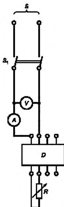
S — источник питания; S_1 — двухполюсный выключатель; V — вольтметр; A — амперметр; D — АВТ; R — переменный резистор
