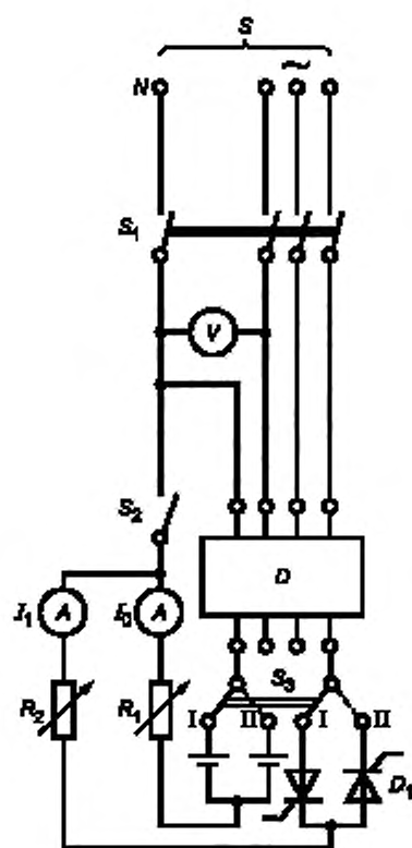
Рисунок 4с — Испытательная цепь для проверки правильности функционирования АВДТ в случае внезапного появления дифференциального пульсирующего постоянного тока с наложением гладкого постоянного дифференциального тока
