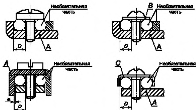
Винтовые выводы
