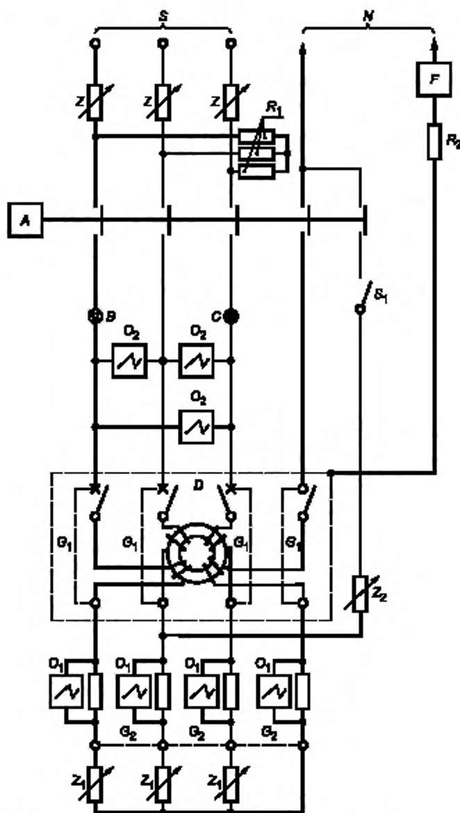
Рисунок 9 — Испытательная цепь для проверки номинальной наибольшей отключающей способности четырехполюсного АВР в трехфазной сети с нейтралью (9.12)
