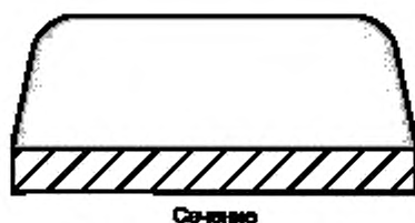
Рисунок 1 — Контур и сечение паяльной пасты: заданное состояние
