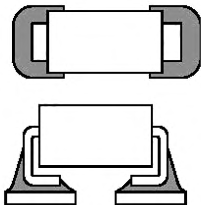
Рисунок А.34 — Смещение: заданное состояние
