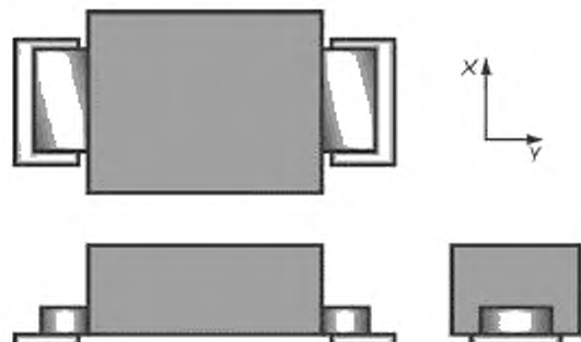
Рисунок 42 — Установка компонента большой мощности с плоскими выступающими выводами: заданное состояние
