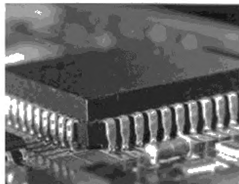
Рисунок А.9 — Галтель припоя: заданное состояние
