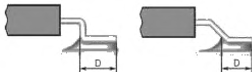
Рисунок А.5 — Галтель припоя: заданное состояние
