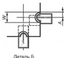
Рисунок 34 — Установка кристаллоносителя: допустимое состояние
