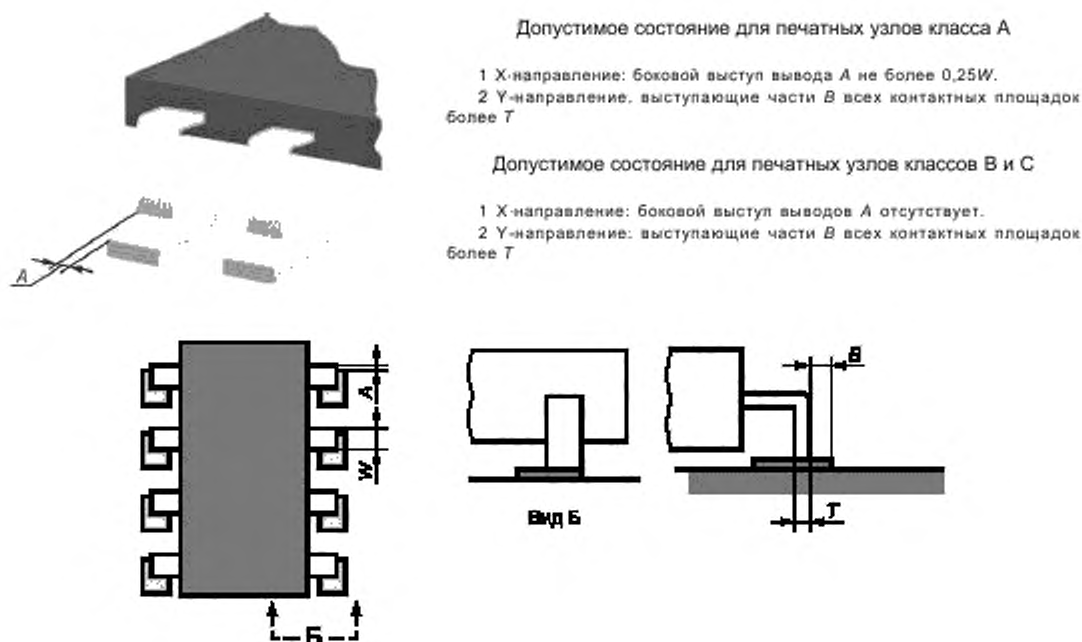
Рисунок 37 — Установка компонента с выводами для пайки встык: допустимое состояние
