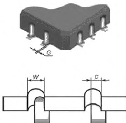
Рисунок А.27 — Галтель припоя: допустимое состояние
