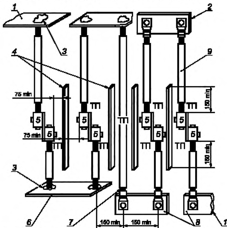
Рисунок L.1 — Испытательное устройство
