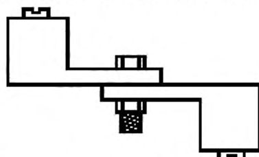
Рисунок L.1 — Испытательное устройство
