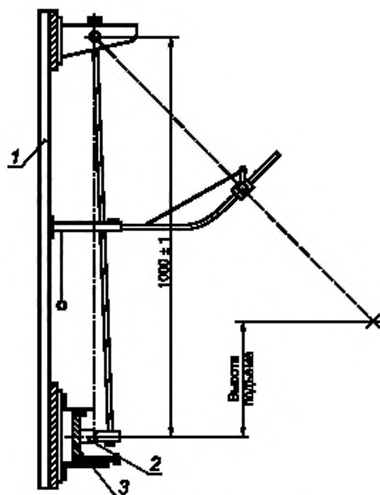
1 — опора, 2 — образец; 3 — монтажная опора
