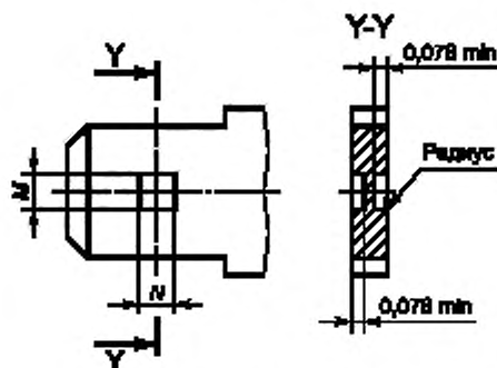
Допуск расположения углубления относительно центральных осей штекера 0,13 мм.
