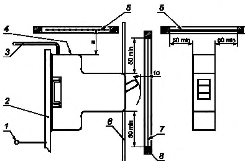
1 — « предохранитель F; 2 — металлическая панель; 3 — кабель; 4 — выхлопное окно; 5 — решетка; 6 — барьер; 7 — полиэтиленовый лист; 8 — рама
