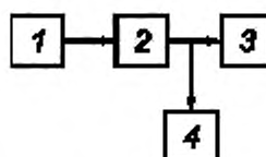
Рисунок 17 — Схема измерения взвешенного шума
