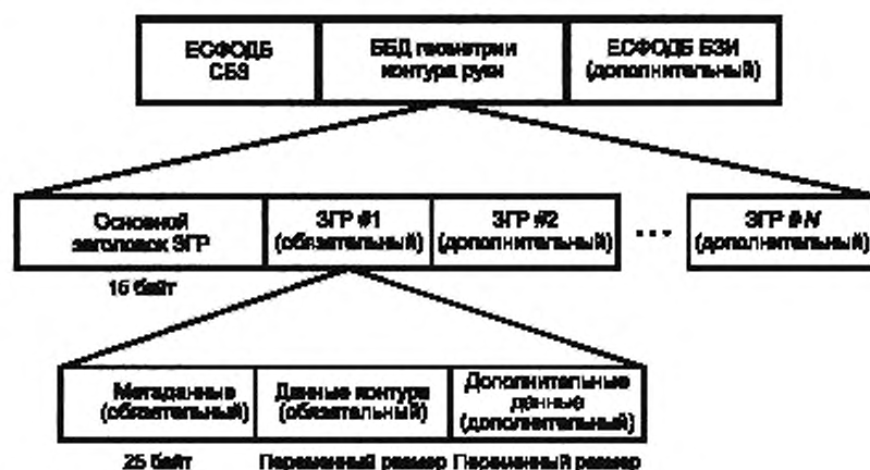
Рисунок 5 — Иерархия элементов ББД
