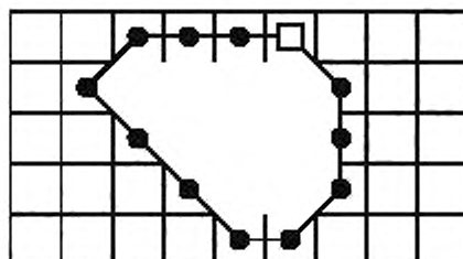
б) 8-связный ЦКФ внешней границы = «4», «4», «4», «0», «7», «7», «7», «0», «1», «2», «2», «3»
