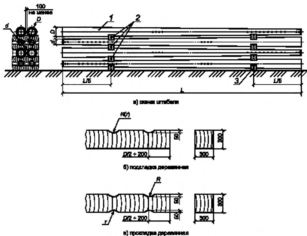
Рисунок Д.1 — Схема хранения стоек железобетонных
