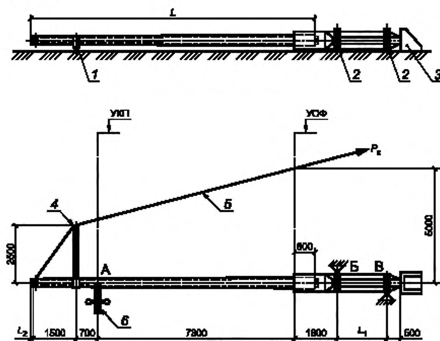
а) стойки СС и СП
