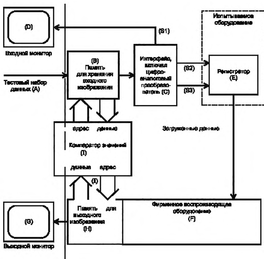
Рисунок 1 — Блок-схема испытаний
