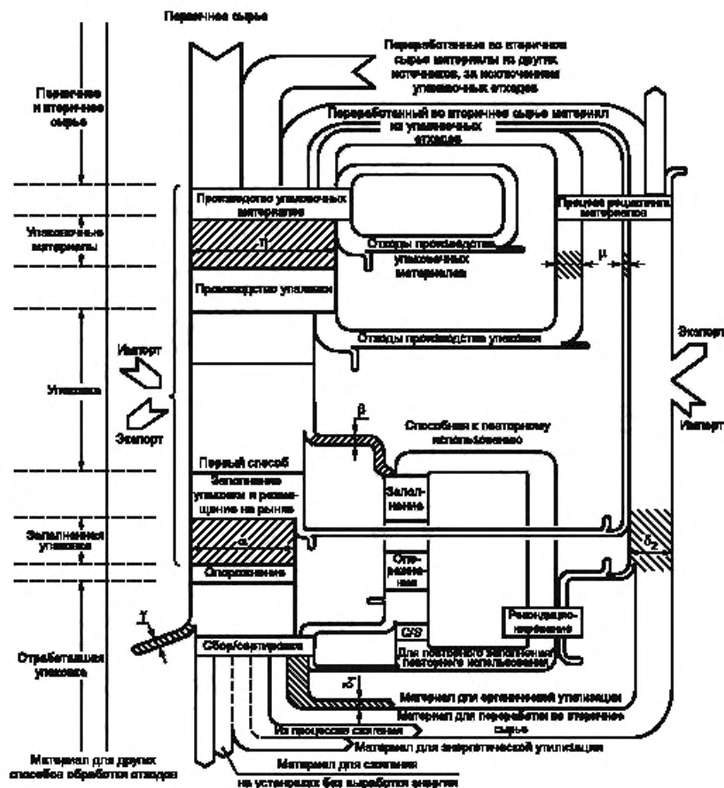
Рисунок 1 — Расчет показателей переработки отработавшей упаковки в качестве вторичных материальных ресурсов по принципу использования пунктов измерения материальных потоков для упаковочных материалов
