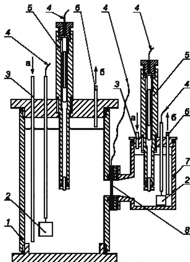
1 — камера наводороживания; 2 — вспомогательный электрод; 3 — трубка для входа инертного газа; 4 — токопровод; 5 — электрод сравнения; 6 — трубка для выхода инертного газа; 7 — окислительная камера; 8 — испытательный образец, а — вход инертного газа; б — выход инертного газа
