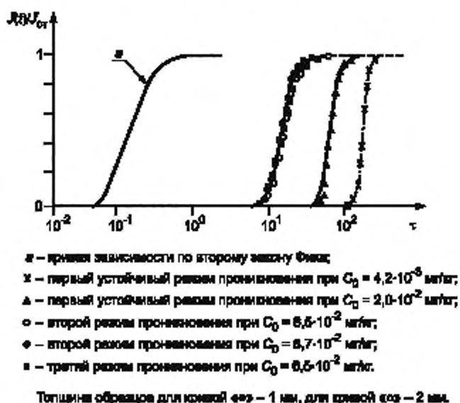
Рисунок 3 — Пример кривых зависимости нормализованных потоков водорода для нержавеющей стали при испытании в растворе хлористого натрия (NaCl) при температуре 77 °C
