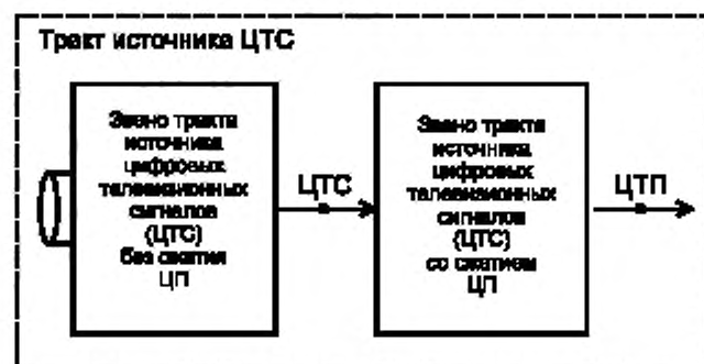
Рисунок 2 — Звенья трасс источника цифровых телевизионных сигналов
