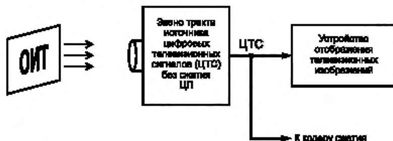
Рисунок 3 — Измерение параметров звена трасс источника цифровых телевизионных сигналов без сжатия цифрового потока
