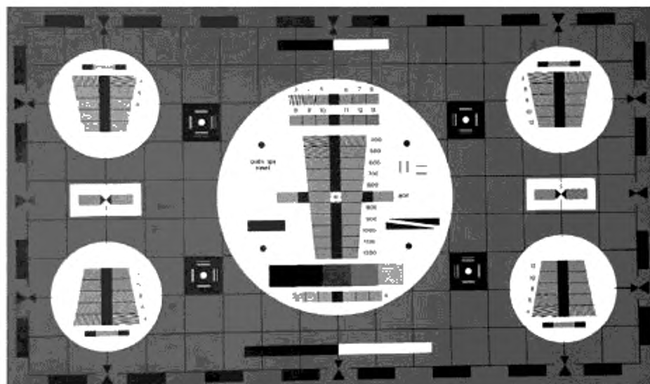
Рисунок А.1 — Оптическая измерительная таблица для измерения глубины модуляции на штриховых мирах и оценки разрешающей способности
