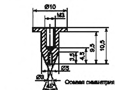
Центральный проводник из латуни. Приблизительно 2:1
