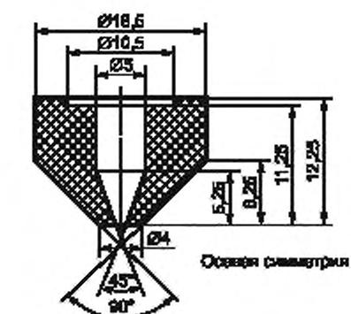
Часть I. Приблизительно 2:1
