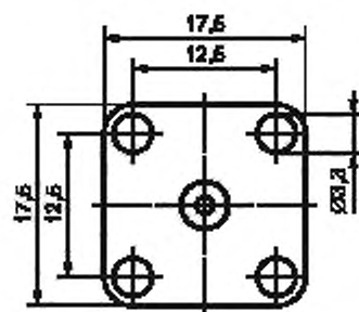
Можно использовать вместо этого соединителя деформированный соединитель N-типа
