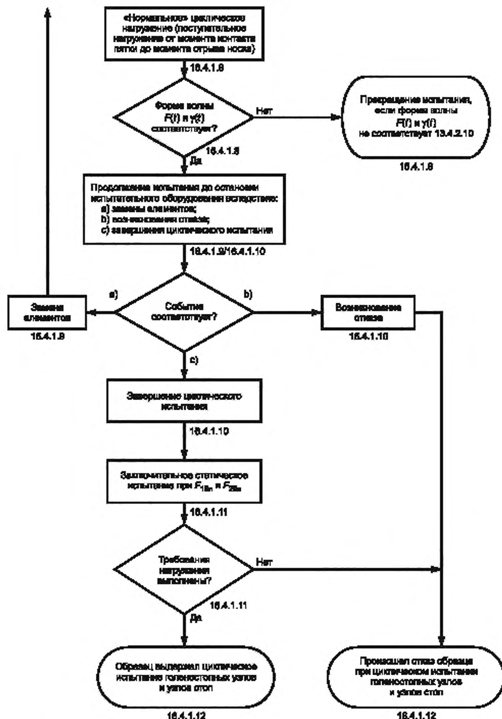
Рисунок 12 — Блок-схема циклического испытания голеноостопных узлов и узлов стоп, установленного в 16.4.1.
