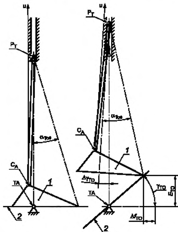
Рисунок Е.3 — Иллюстрация влияния A - P смещения \Delta f на угловое перемещение \Delta f образца относительно верхней точки приложения нагрузки P_T
