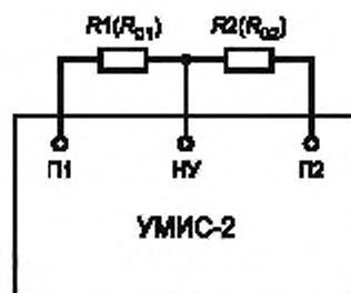
Рисунок 5 — Схема поверки делителя напряжения методом измерения отношения сопротивлений
