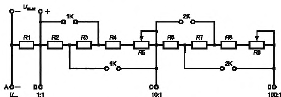
U_{вх} — входное напряжение; U_{вых} — выходное напряжение; A, B, C, D — клеммы подключения; R1-R4, R6-R8 — постоянные резисторы, R5, R9 — резисторы подстройки; 1K, 2K — контакты переключателя
