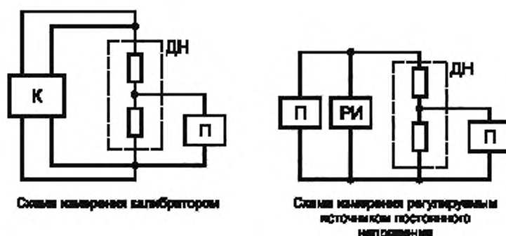
ДН — делитель напряжения; К — эталонная мера постоянного напряжения (калибратор); РИ — регулируемый источник постоянного напряжения; П — эталонное средство измерения постоянного напряжения
