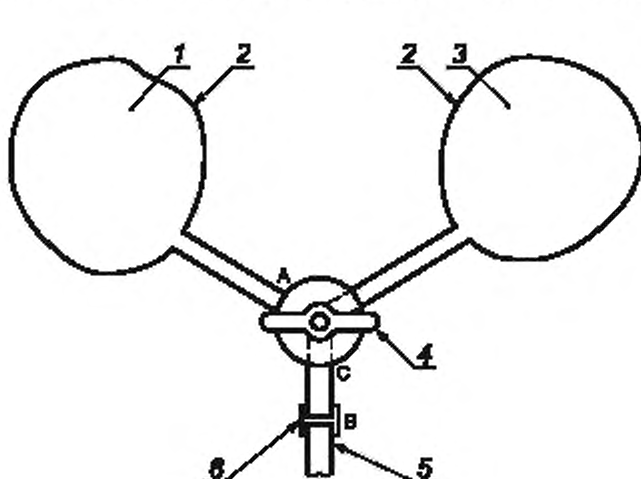
1 — ПГС; 2 — газовые емкости; 3 — чистый воздух; 4 — двухходовой кран; 5 — преобразовательный зонд или газовый вход прибора; 6 — устройство для подключения прибора
