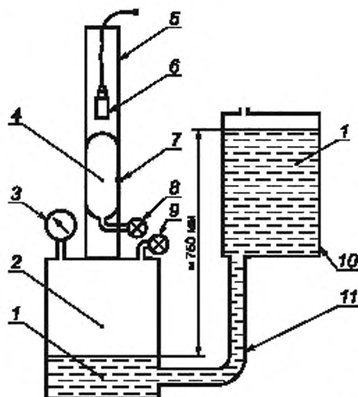
Рисунок В.6 — Схема установки, обеспечивающей скачкообразный переход из чистого воздуха в газозелоздушную смесь
