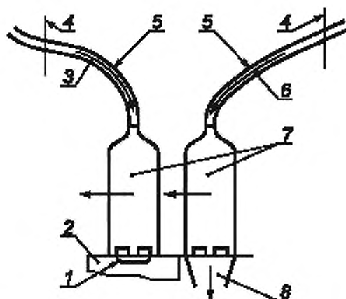
1 — вход газонализатора (датчика); 2 — газонализатор (датчик); 3 — чистый воздух; 4 — расходомер; 5 — гибкая трубка; 6 — ПГС; 7 — идентичные трубчатые аппликаторы; 8 — сброс газа
