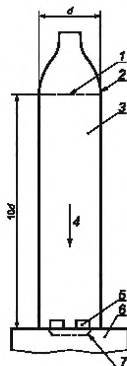
1 — диффузионный барьер; 2 — расширение аппликатора; 3 — трубчатый аппликатор; 4 — поток чистого воздуха; 5 — выемка; 6 — газонализатор или выносной датчик; 7 — вход газонализатора или выносного датчика
