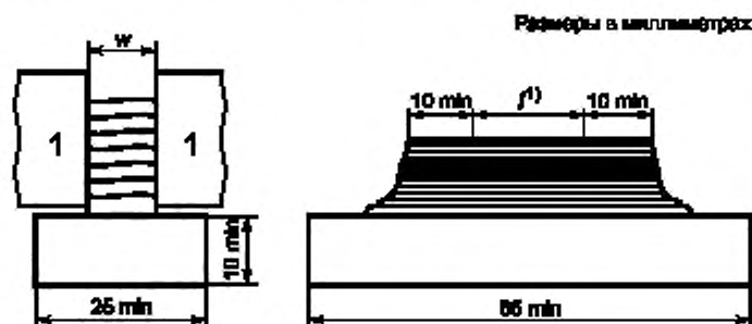
Медный брусок 70 × 25 × 25 мм
