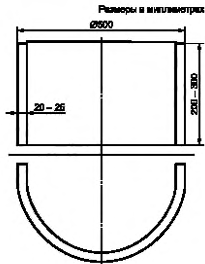
Рисунок 3 — Центробежнолитая трубная заготовка для изготовления СО СФФ
