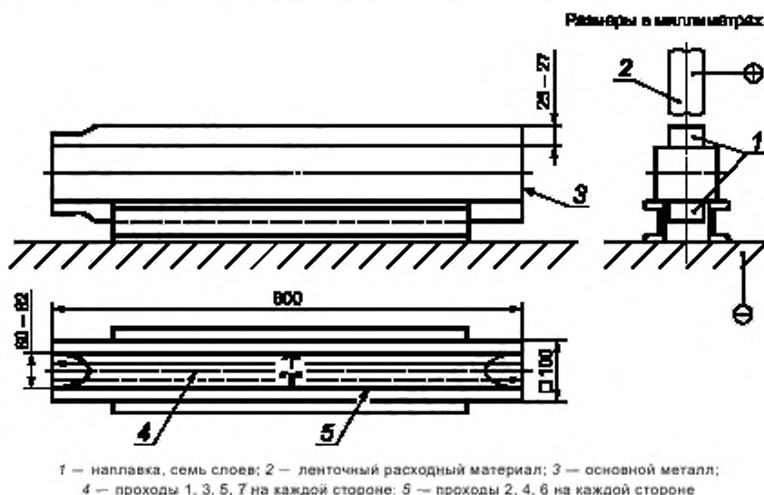
Рисунок А.1 — Метод получения наплавленного металла для вторичных стандартных образцов с помощью ленточных электродов
