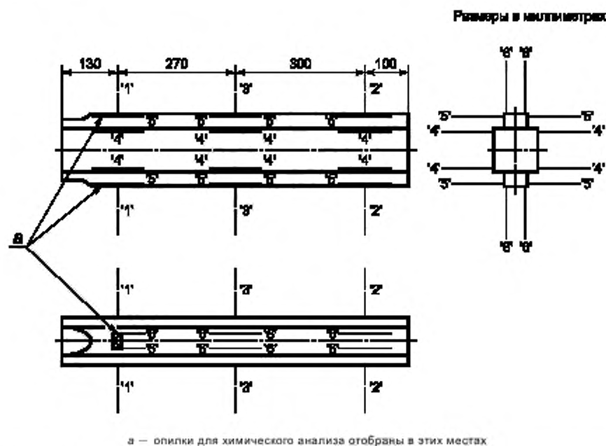
Рисунок А.3 — Последовательность обрезки для вторичного стандарта плакировкой лентой
