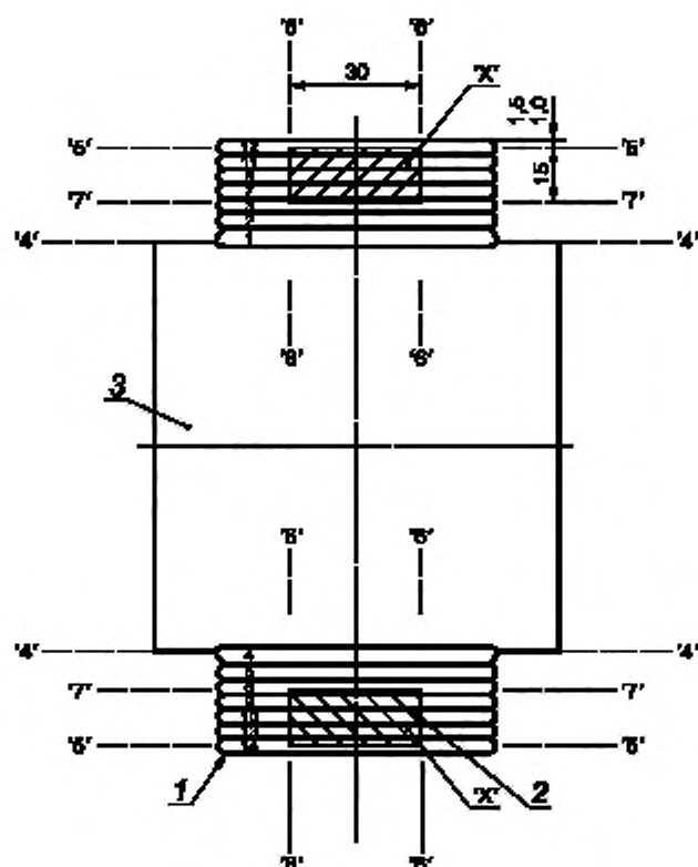
Рисунок А.2 — Последовательность выполнения наплавки при использовании ленточных электродов и вырезки вторичных стандартных образцов
