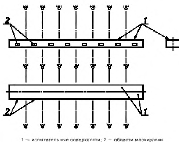
Рисунок А.4 — Выделение отдельных ленточных плакировок вторичных стандартов
