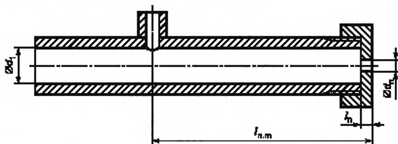
Рисунок 1 — Конфигурация сопла
