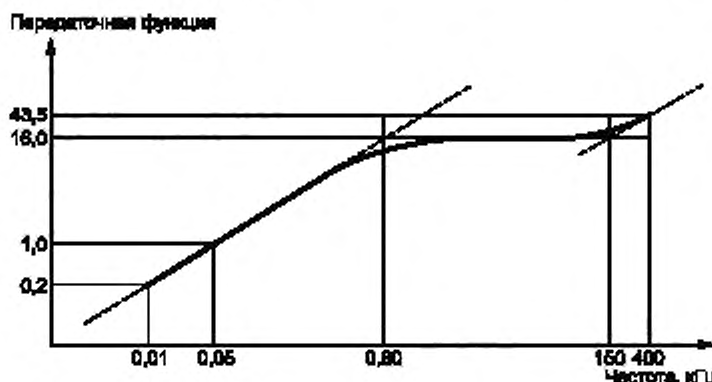
Рисунок 1 — Передаточная функция
