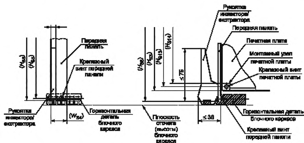
Деталь X
