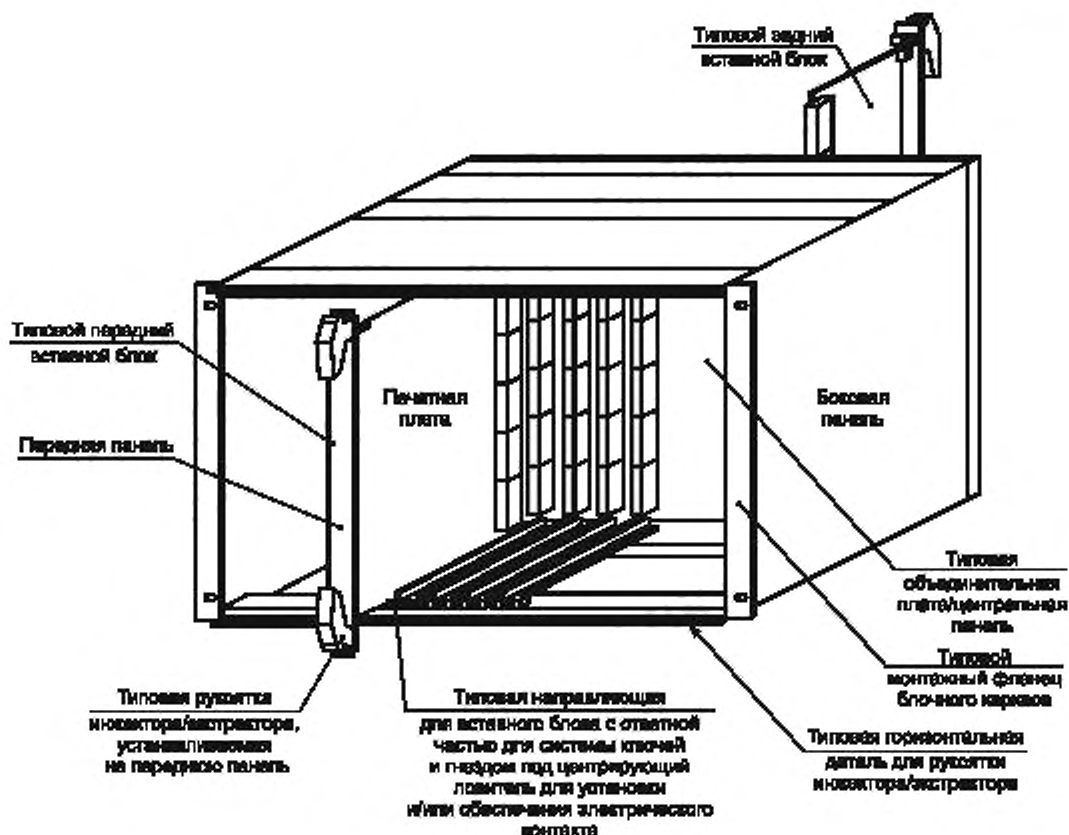
Рисунок 3 — Общая компоновка
