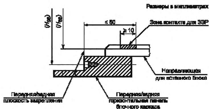
Рисунок 21 — Размеры блочного каркаса. Контактные элементы для ЗЭР на направляющих вставного блока
