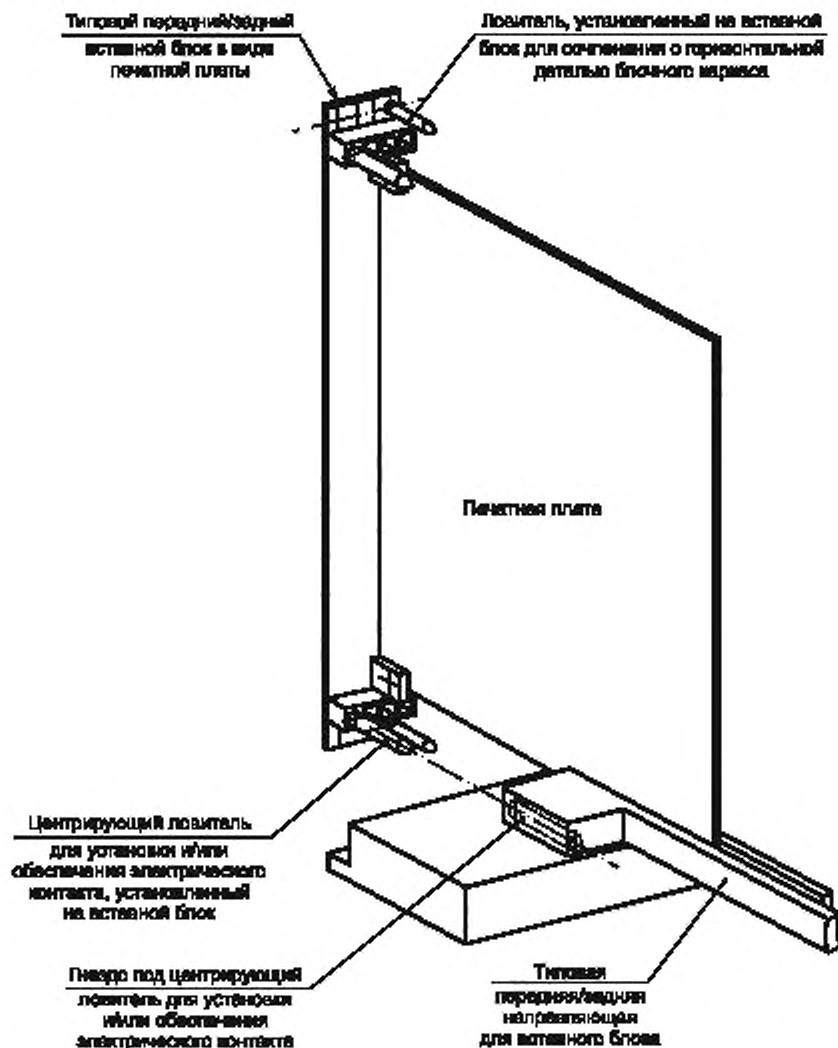
Рисунок 16 — Компонента системы центрирующего ловителя для блочных каркасов и вставных блоков
