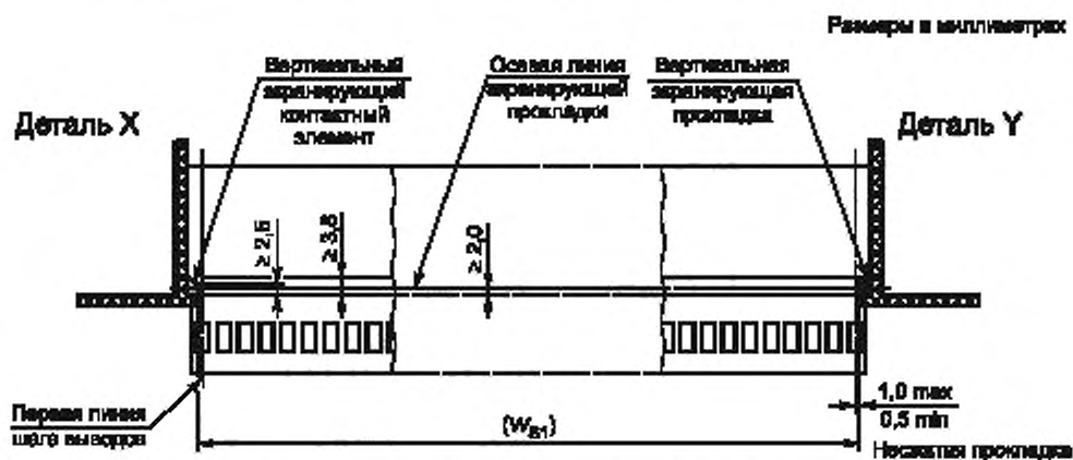
Рисунок 8 — Размеры блочного каркаса. Средства электромагнитного экранирования
