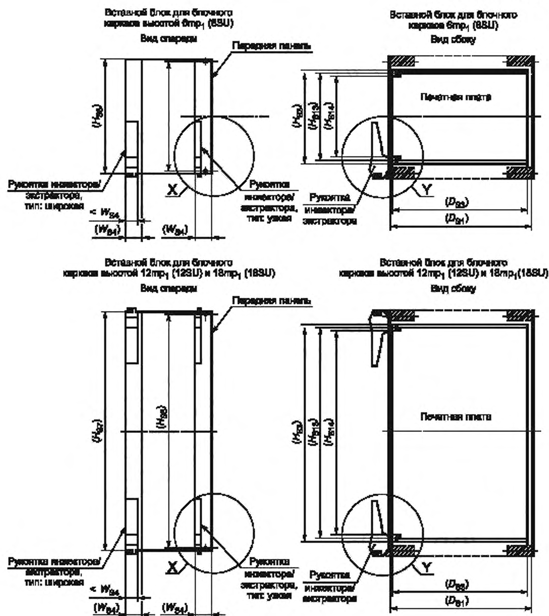
Рисунок 6 — Размеры вставных блоков, рукоятки инжектора/экстрактора для вставных блоков
