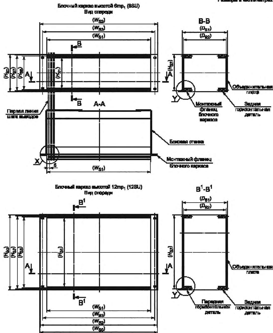
Рисунок 4 — Размеры блочного каркаса для рукоятки инжектора/экстрактора вставных блоков
