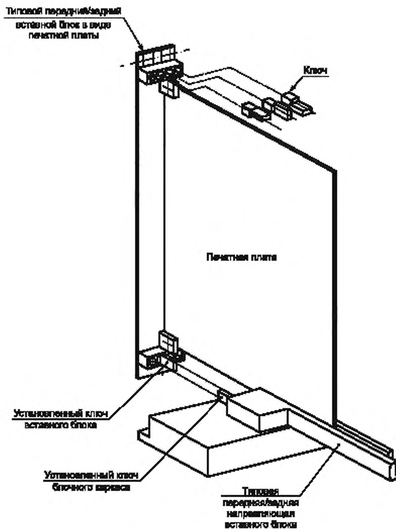
Рисунок 11 — Компоненты системы ключей кодирования для вставных блоков
