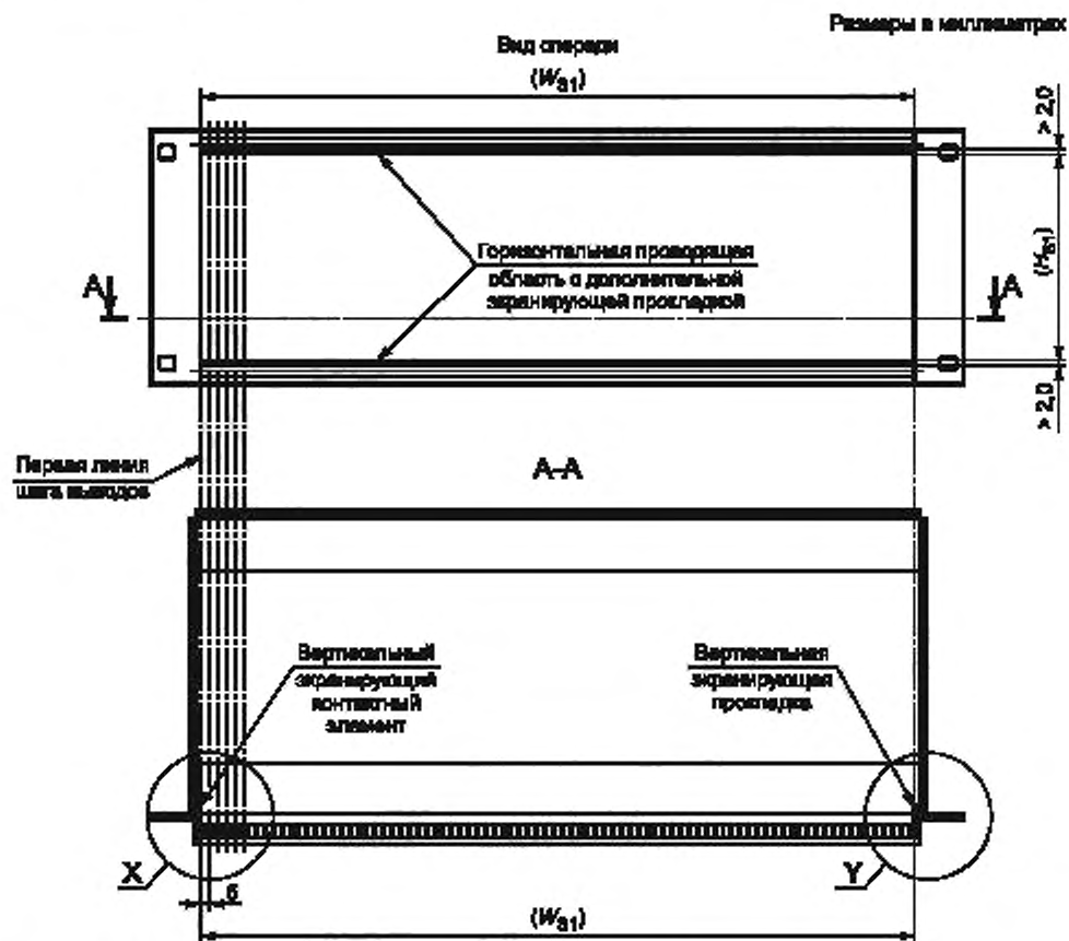
Рисунок 8 — Размеры блочного каркаса. Средства электромагнитного экранирования
