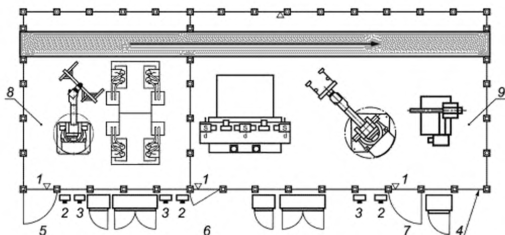
1 — блокировка подхода; 2 — переустановка; 3 — аварийная остановка; 4 — предохранение по периметру; 5 — доступ закрыт; 6 — доступ открыт
