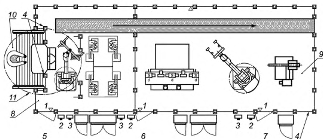
1 — блокировка прохода; 2 — аварийная остановка; 3 — переустановка; 4 — предохранение по периметру; 5 — доступ закрыт; 6 — доступ закрыт; 7 — доступ закрыт; 8 — зона А; 9 — зона В; 10 — зона С; 11 — сенсорное устройство постоянного обнаружения присутствия
