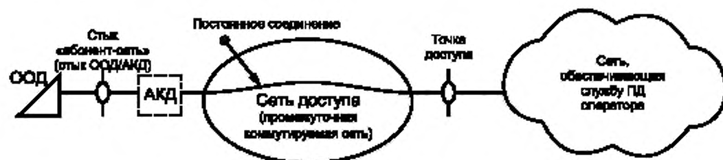
в) непрямой доступ с постоянным соединением
