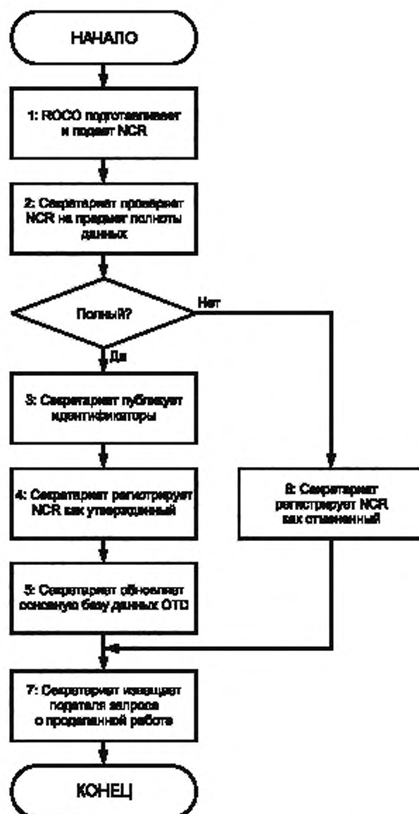
Рисунок 2 — Процедура добавления концепции
