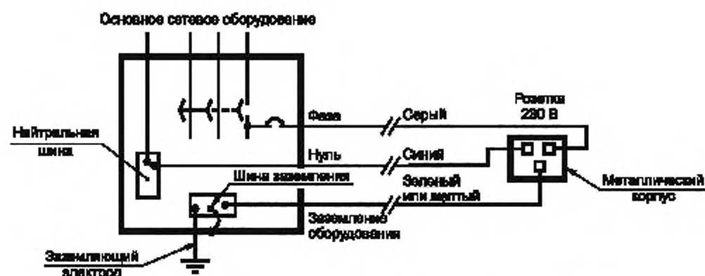
Рисунок 4в — Пример энергосистемы Великобритании — Однофазная система
