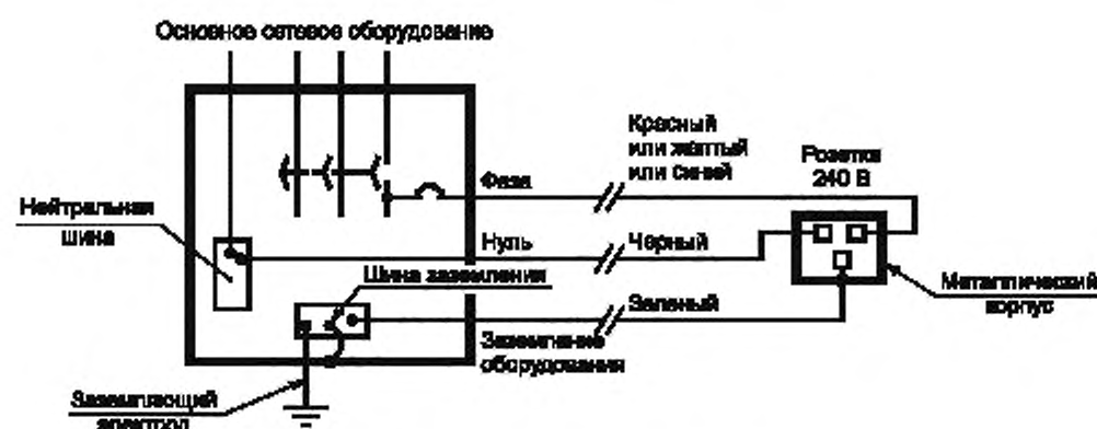
Рисунок 4б — Пример Малайзийской энергосистемы
