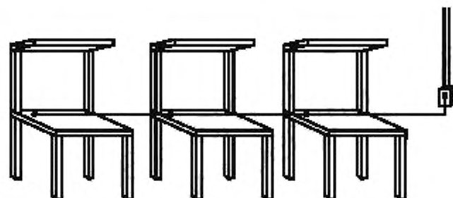
Рисунок 6 — Пример нерекондуемого заземления последовательно соединенных столов
