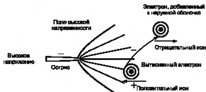
Рисунок 11 — Коронная ионизация — отрицательная
