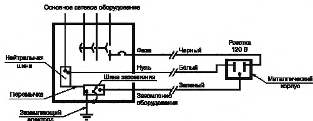
Рисунок 4а — Пример Североамериканской энергосистемы
