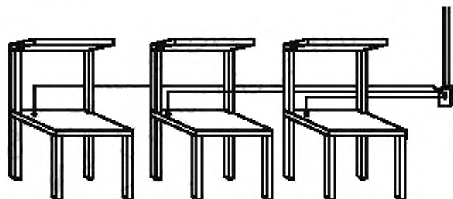
Рисунок 5 — Пример рекомендуемого индивидуального заземления столов
