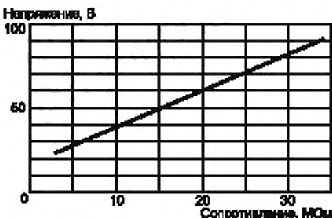
Рисунок 7 — Зависимость между напряжением тела и сопротивлением относительно земли
