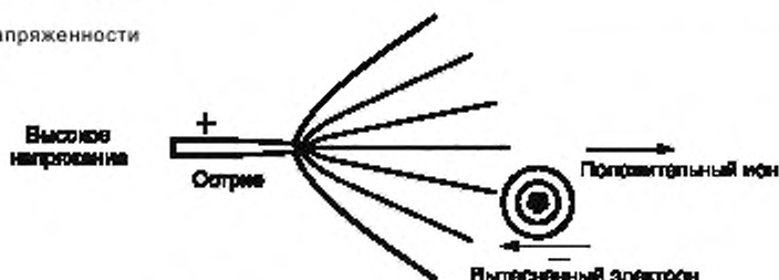
Рисунок 10 — Коронная ионизация — положительная
