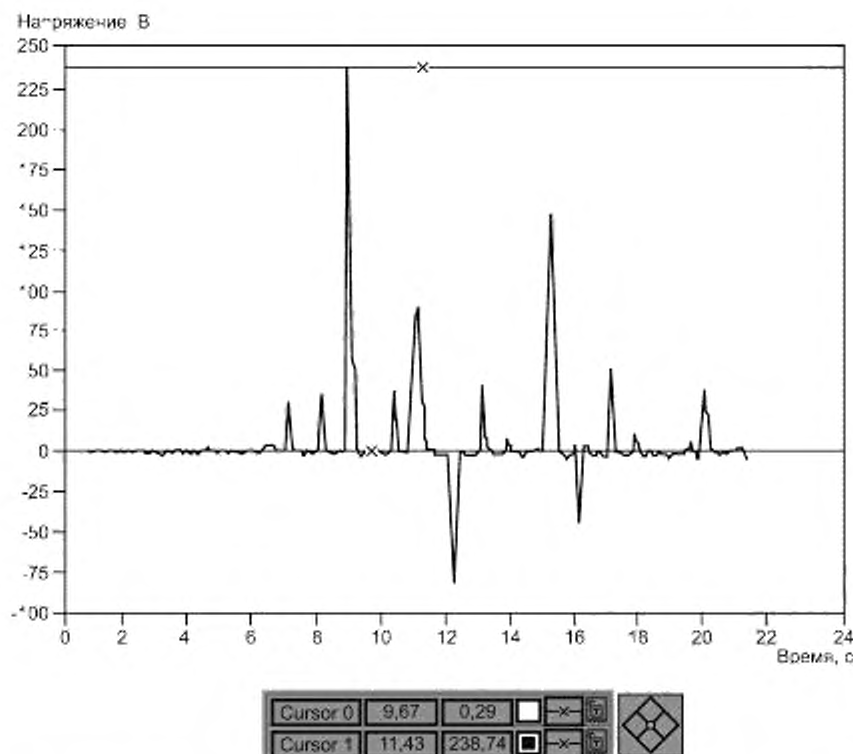
Рисунок 6 — Напряжение на сотруднике, идущем по заземленному проводящему полу с двумя надетыми ремешками заземления
