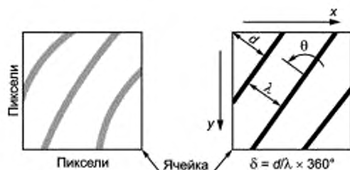
Рисунок 3 — Представление спектральных составляющих ячейки изображения отпечатка пальца
