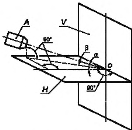
Рисунок 2 — Стенд для испытания приборов типа C 11
