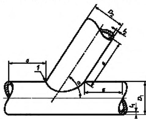
1 — подготовка и сборка соединения, как описано в pWPS; a — минимальное значение 150 мм; D_1 — наружный диаметр трубы, мм; D_2 — наружный диаметр отвода; t_1 — толщина материала основной трубы; t_2 — толщина материала отвода; \alpha — угол отвода
