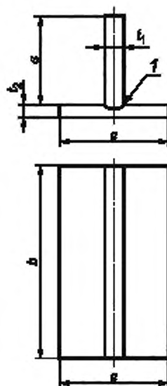
1 — сварной шов с одной или с обеих сторон, подготовка и сборка соединения, как описано в pWPS; a — минимальное значение 150 мм; b — минимальное значение 350 мм; t — толщина материала
