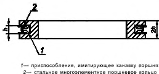
Рисунок 18 — Схема приспособления для контроля компрессионных и маслосъемных колец в сборе
