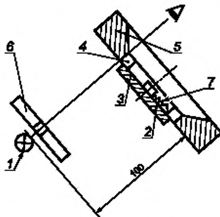
1 — источник света; 2 — непрозрачный экран; 3 — образец просвета; 4 — контролируемое кольцо; 5 — гладкий кольцевой калибр; 6 — фильтр; 7 — имитатор расширителя (расширитель применять только при контроле колец, работающих с расширителем)
