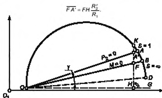
Рисунок 5.4.2 — Построение окружностей тока для двигателей с фазным ротором
