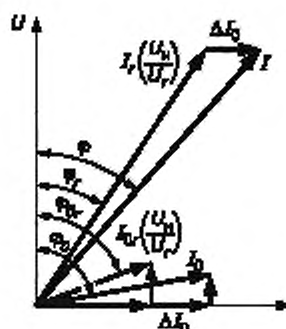
Рисунок 4 — Векторная диаграмма для определения тока статора
