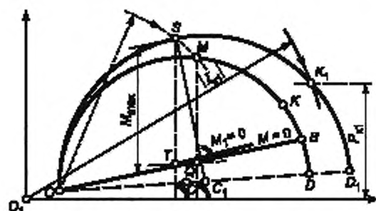
Рисунок Б.7.1 — Определение максимального момента для короткозамкнутых двигателей и двигателей с фазным ротором
