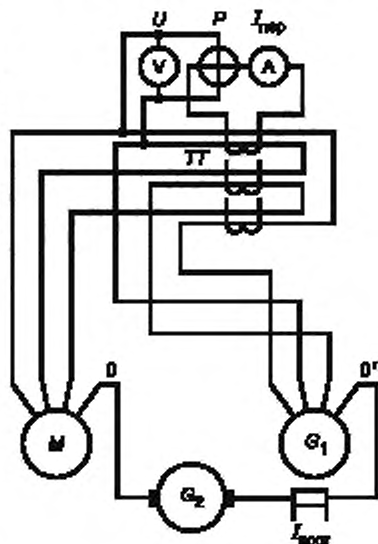
M — испытуемый двигатель; G_1 — источник питания переменного тока; G_2 — источник питания постоянного тока; \emptyset, \emptyset' — нулевые выводы обмотки; TT — трансформаторы тока
