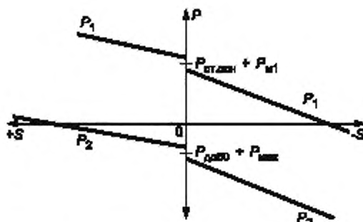
Рисунок 9 — Определение добавочных потерь холостого хода
