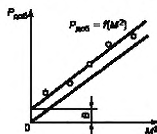
Рисунок 10 — Определение добавочных потерь методом непосредственной нагрузки
