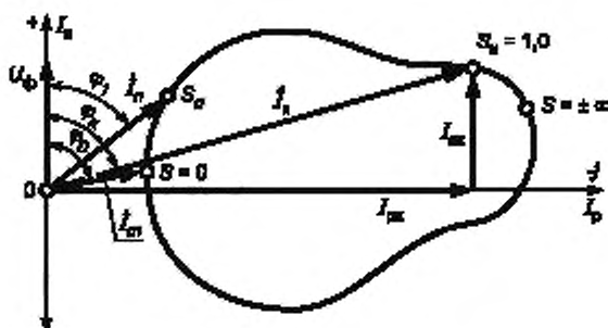
Рисунок 7 — Частотная характеристика асинхронного двигателя
