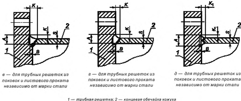
Рисунок 1 — Узел соединения трубной решетки с кожухом (Лист 2)
