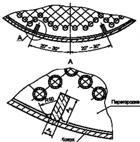
Рисунок 3 — Расположение полос скольжения в трубных пучках аппаратов
