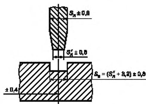
Рисунок 8 — Узел соединения перегородки с решеткой
