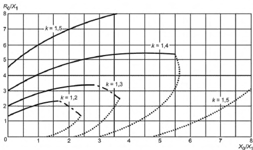
Рисунок А.4 — Соотношение между R_0 / X_1 и X_0 / X_1 для постоянных значений коэффициента замыкания на землю k , где R_1 = X_1
