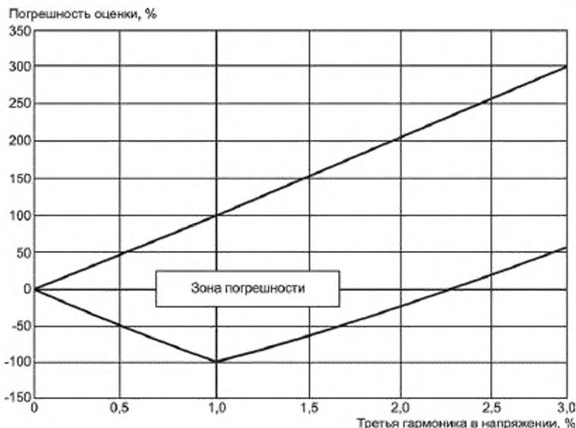
Рисунок 10 — Ошибка в оценке третьей гармоники тока утечки для различных фазовых углов третьей гармоники напряжения сети при учете различных емкостей и вольтамперных характеристик нелинейных металлооксидных резисторов
