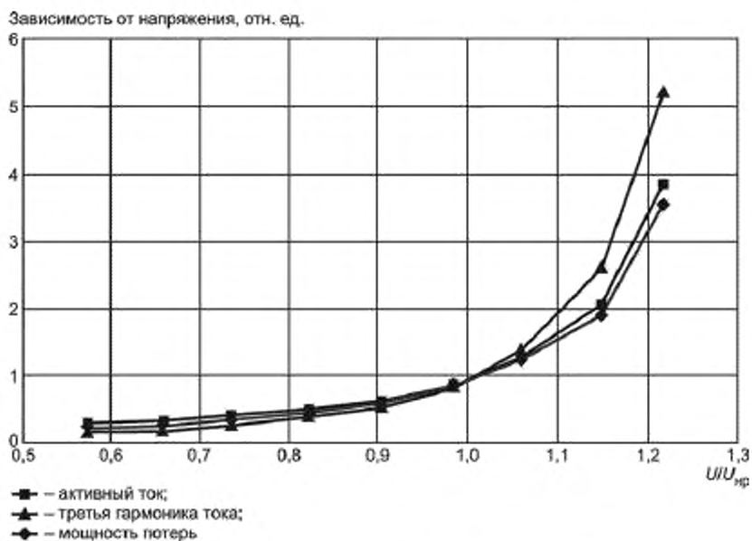
Рисунок 6 — Типичная нормализованная зависимость от напряжения при температуре +20 °C
