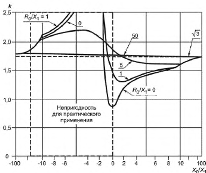
Рисунок А.1 — Коэффициент замыкания на землю k на основе X_0/X_1 , для R_1/X_1 = R = 0
