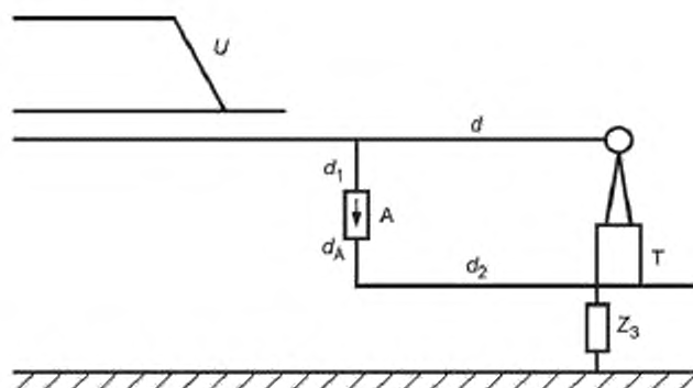
Рисунок 2а — Установки без контура заземления (распределительные сети)
