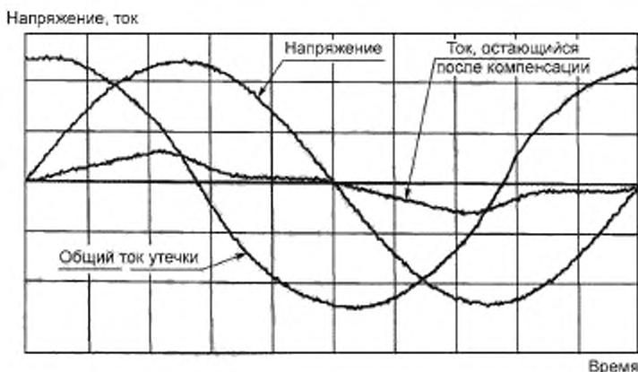
Рисунок 9 — Ток, остающийся после компенсации емкостного тока, при U_{нр}
