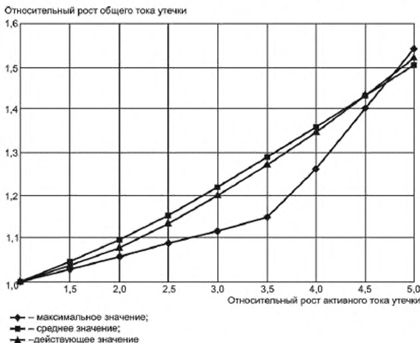
Рисунок 8 — Влияние роста активного тока утечки на рост полного тока утечки
