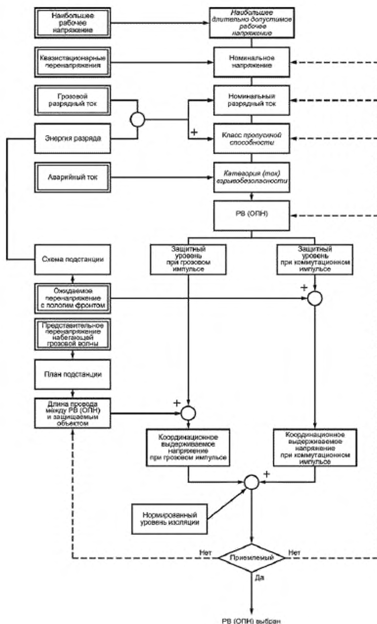
Рисунок 1 — Структурная схема выбора РВ (ОПН)
