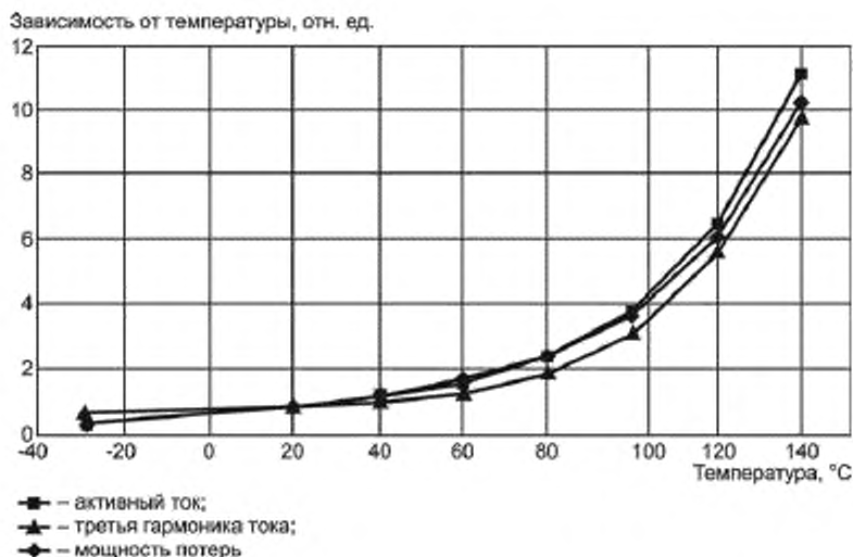
Рисунок 7 — Типичная нормализованная зависимость от температуры при наибольшем длительно допустимом рабочем напряжении U_{\text{нр}}
