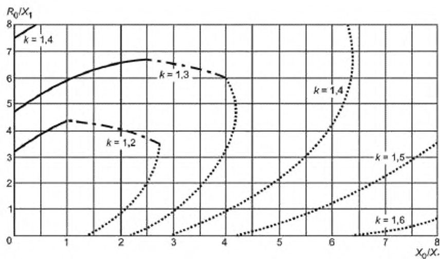
Рисунок А.5 — Соотношение между R_0 / X_1 и X_0 / X_1 для постоянных значений коэффициента замыкания на землю k , где R_1 = 2X_1
