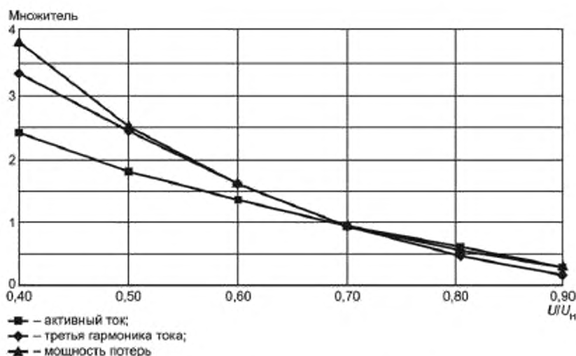
Рисунок 11 — Типичная информация для приведения к условиям «стандартного» рабочего напряжения
