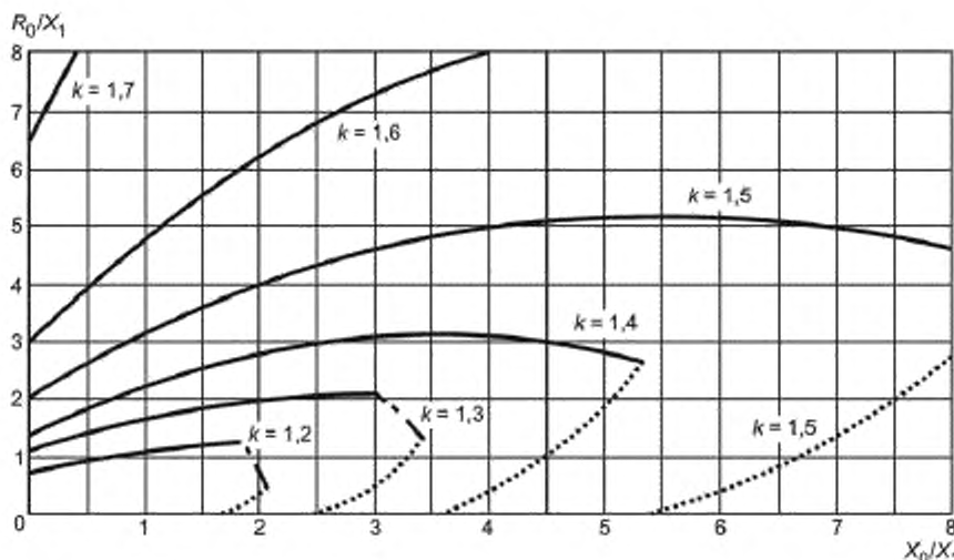
Рисунок А.3 — Соотношение между R_0/X_1 и X_0/X_1 для постоянных значений коэффициента замыкания на землю k , где R_1 = 0.5X_1
