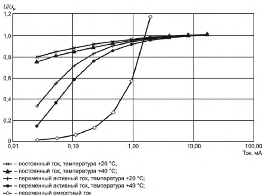
Рисунок 5 — Типичные вольтамперные характеристики нелинейных металлооксидных резисторов
