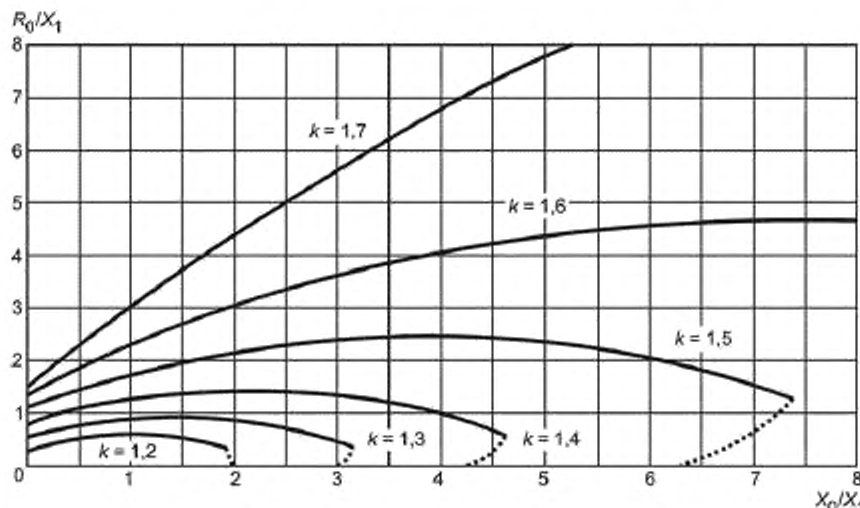
Рисунок А.2 — Соотношение между R_0/X_1 и X_0/X_1 для постоянных значений коэффициента замыкания на землю k , где R_1 = 0
