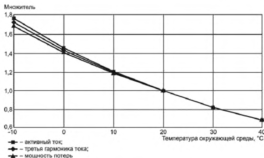
Рисунок 12 — Типичная информация для приведения к условиям «стандартной» температуры окружающей среды
