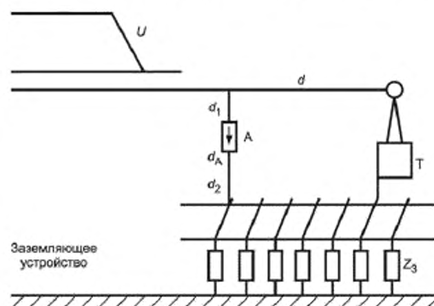
Рисунок 2б — Установки с контуром заземления (подстанции)
