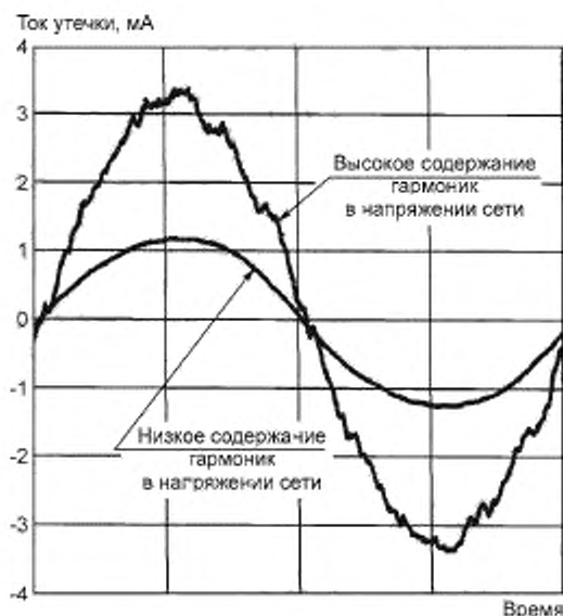
Рисунок 4 — Типичный ток утечки ОПН в условиях эксплуатации
