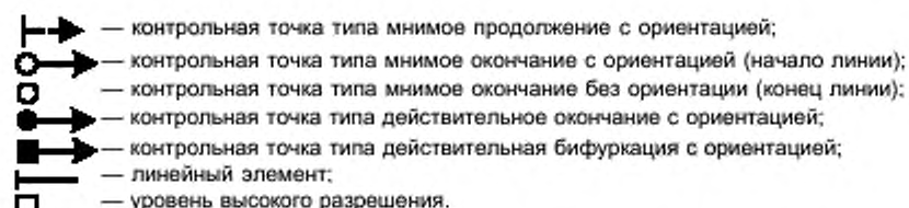
Рисунок А.1 — Элементы кодирования контрольной точки
