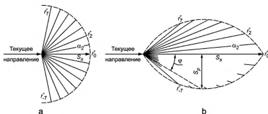
а — при S_s=0 используется постоянная длина шага. В данном случае при угловом разрешении 11,25^\circ ; б — при S_s>0 шаги малых углов изгиба увеличиваются в то время, как уменьшаются шаги больших углов. В данном случае 15 направлений закодировано при высоком угловом разрешении 5,625^\circ .
