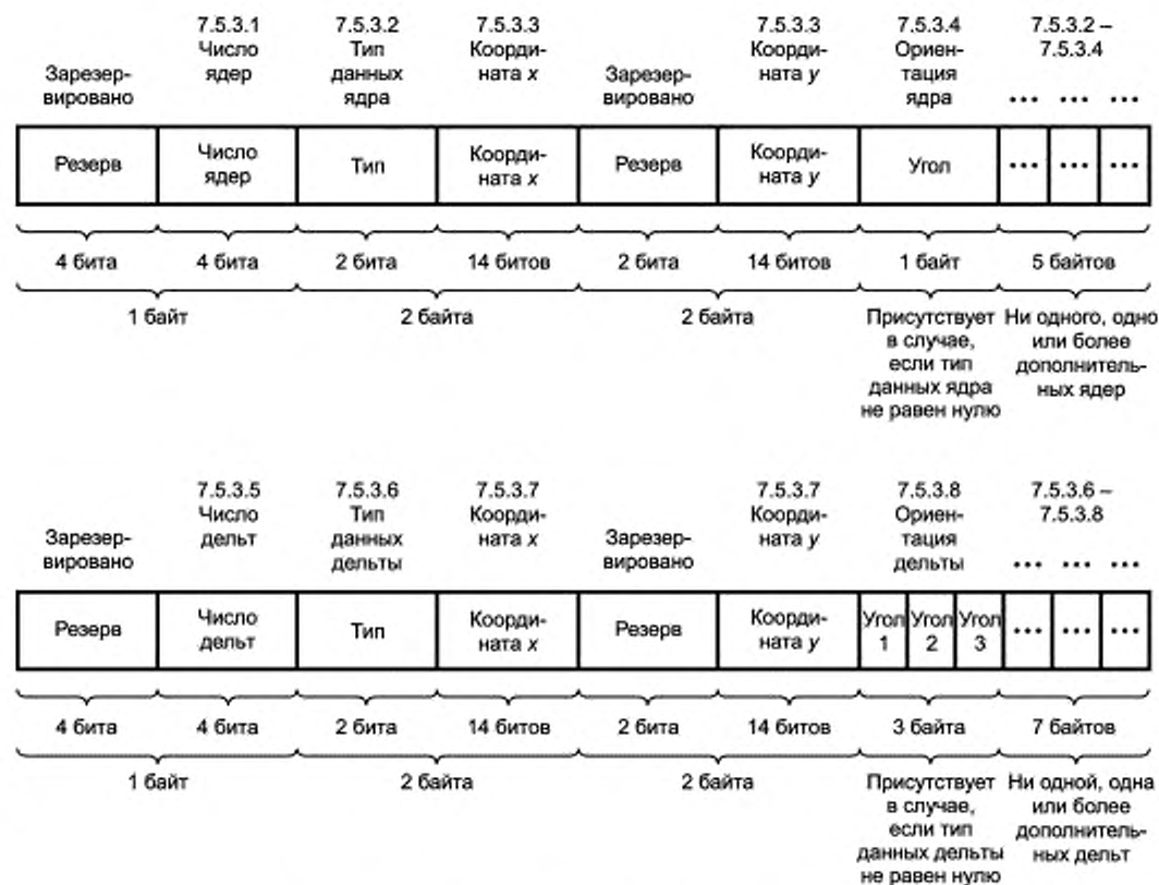
Рисунок 8 — Структура формата данных ядра и дельты
