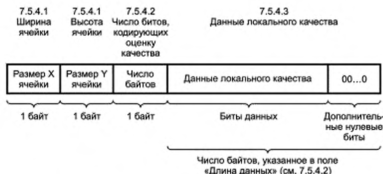
Рисунок 9 — Структура формата данных локального качества
