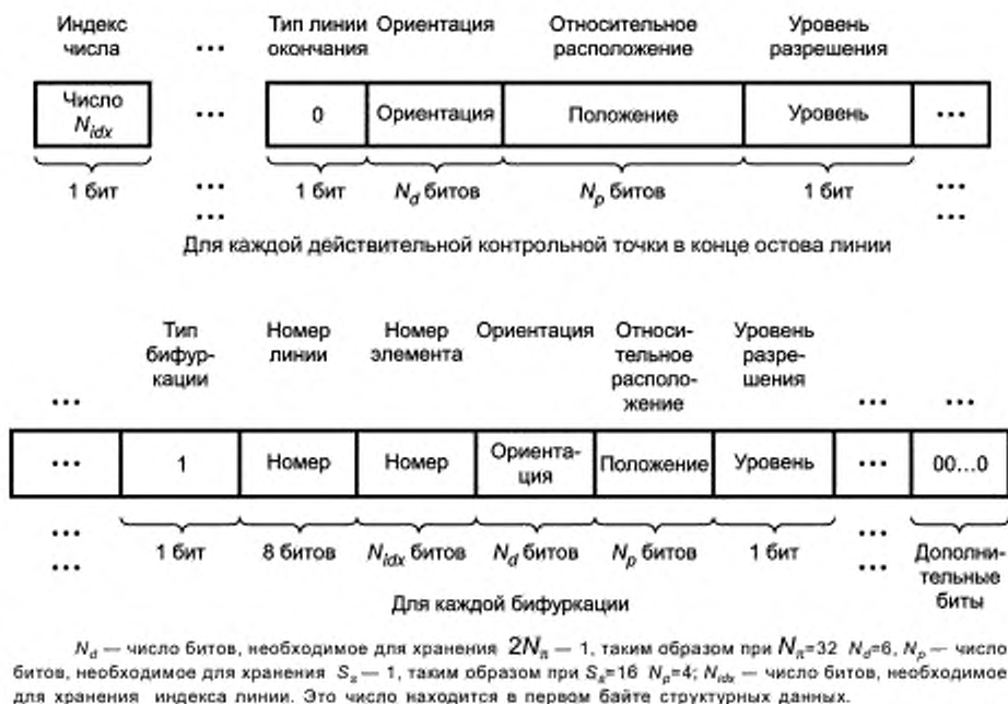
Рисунок 12 — Структура формата данных отпечатка пальца
