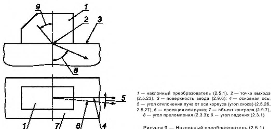
Рисунок 9 — Наклонный преобразователь (2.5.1)
