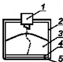
а) прямой преобразователь (2.5.17) (для контактного метода контроля)
