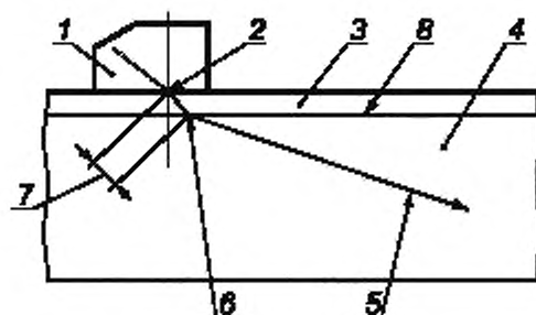
1 — наклонный преобразователь (2.5.1); 2 — точка выхода (2.5.23); 3 — контактная среда (2.10.1); 4 — объект контроля (2.9.7); 5 — ось пучка (2.1.7); 6 — точка ввода (2.9.2); 7 — путь, пройденный в контактной среде (2.10.3); 8 — поверхность ввода (2.9.6)
