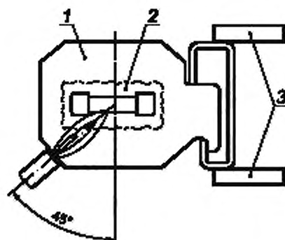
1 — колодка выводов для плавких предохранителей; 2 — часть колодки в области выводного зажима; 3 — фиксирующие части
