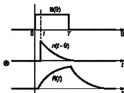
Рисунок BB.4 — Значение ответа R(t) , произведенного скручиванием прямоугольного стимула dB/dt , и функции ответа импульса нерва n(t - \theta)
