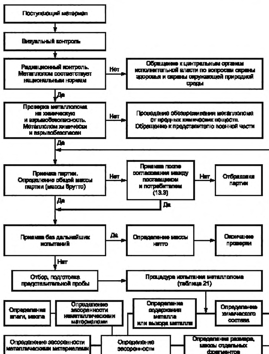
Рисунок 1 — Схема проверки поступающего металлолома
