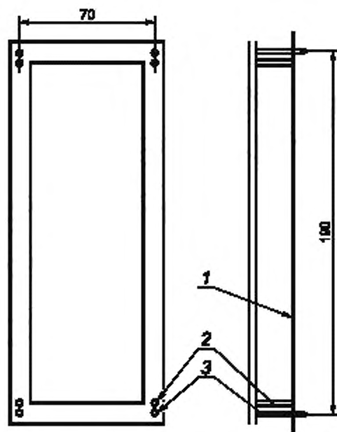
1 — образец для испытаний; 2 — разделительная ножка; 3 — палец крепления
