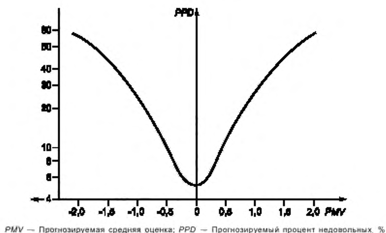
Рисунок 1 — PPD как функция PMV
